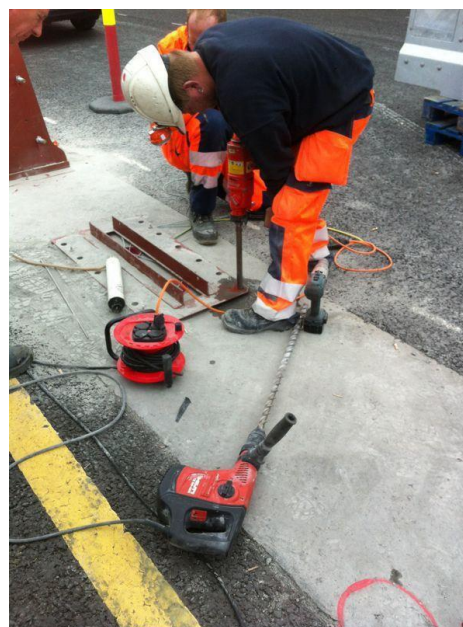
Vŕtanie kotiev pre rámy priechodu CADO
